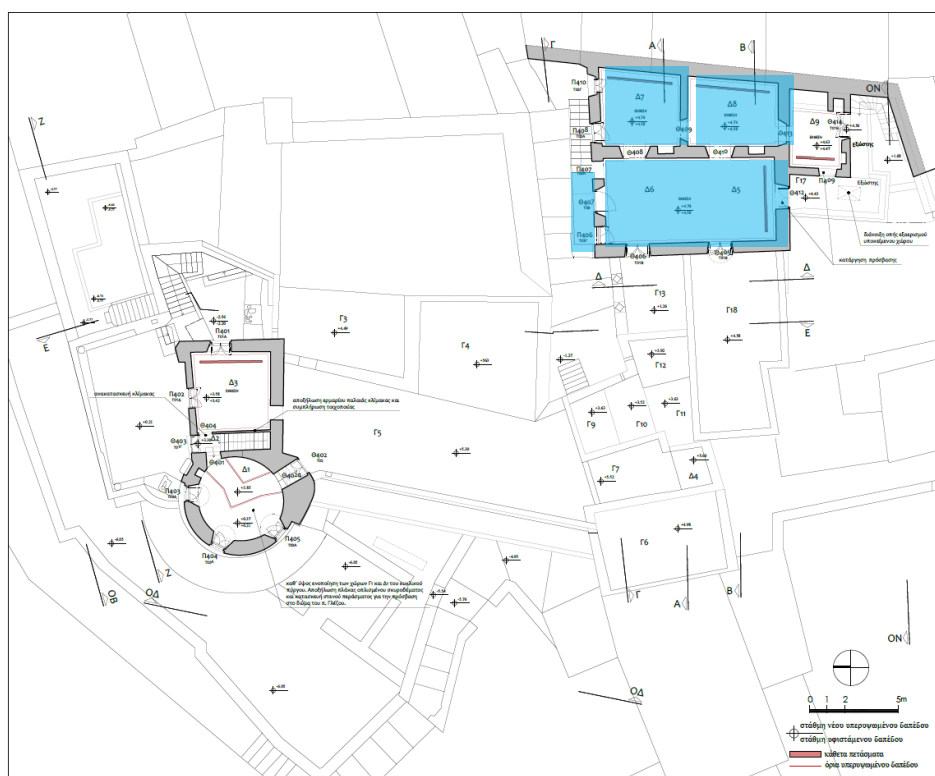
Σχ.5: Κάτοψη χώρων Δ' στάθμης Πύργου-Γλέζου Αεροπορίας, όπου απαιτείται προμήθεια κόντρα πλακέ πατωμάτων.
