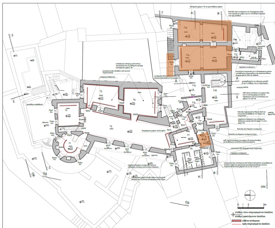
Σχ.4: Κάτοψη χώρων Γ' στάθμης Πύργου-Γλέζου Αεροπορίας, όπου απαιτείται προμήθεια σανίδων οροφών.
