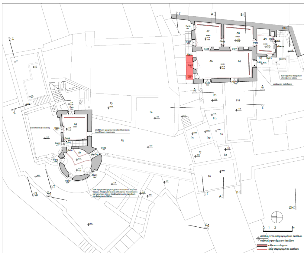
Σχ.6: Κάτοψη χώρων Δ' στάθμης Πύργου-Γλέζου Αεροπορίας, όπου απαιτείται προμήθεια σανίδων δαπέδου.
