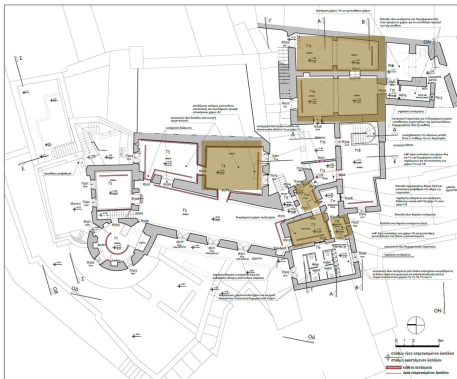
Σχ.3: Κάτοψη χώρων Γ' στάθμης Πύργου-Γλέζου Αεροπορίας, όπου απαιτείται προμήθεια δομικής ξυλείας.
